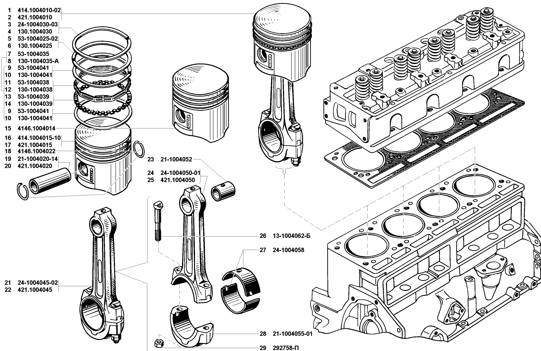
Рис. 5. Поршень и шатун (1004) Fig. 5. Piston and connecting rod (1004)
